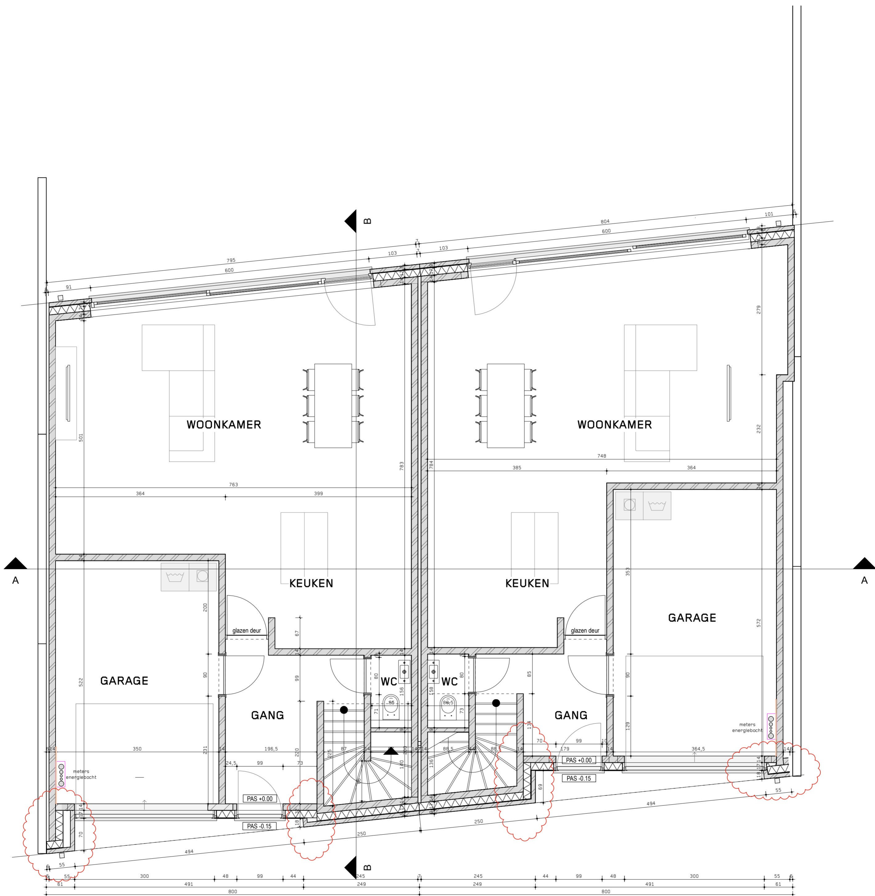
nieuwe toestand - N100 (A4) Schaal: 1:50
